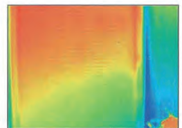
Thermografische Aufnahmen an isolierverglastem Fenster mit Duette®.
